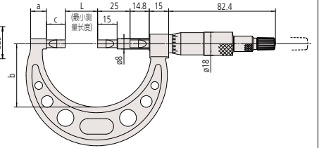
测量范围小于 50mm 普通型
