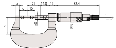
测量范围小于 50mm 普通型
