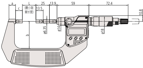
测量范围小于 50mm 数显型 BLM-25MX ~ 50MX
