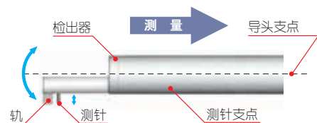
有轨阶差测量示例
